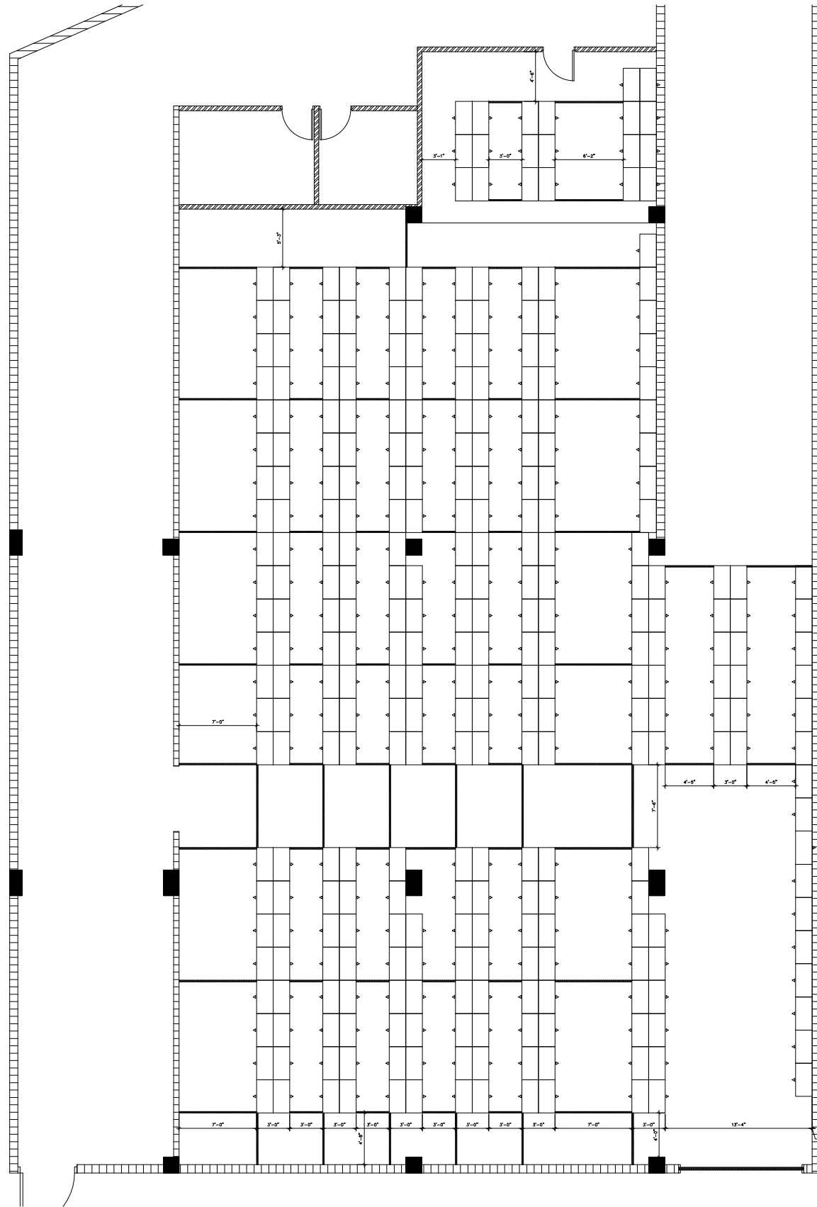
DISTRIBUCIÓN DE ANAQUELES ESCALA: 3/16" = 1'-0"
